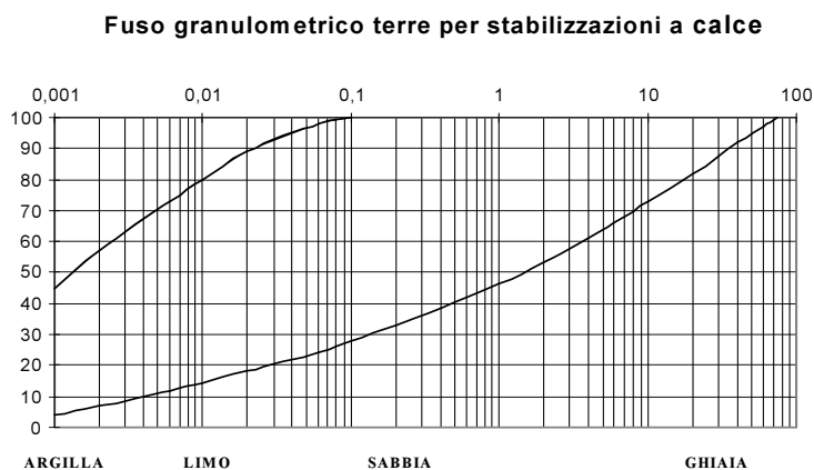
Fig.2.1 Fuso granulometrico di riferimento (CNR-B.U. n° 36)
